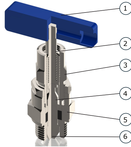
Fig 2. Partes de bonete.
